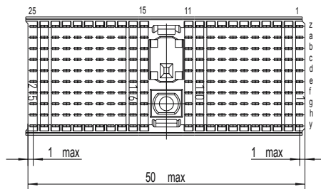
Lochbild fuer Leiterplatte (Bestueckungsseite)
