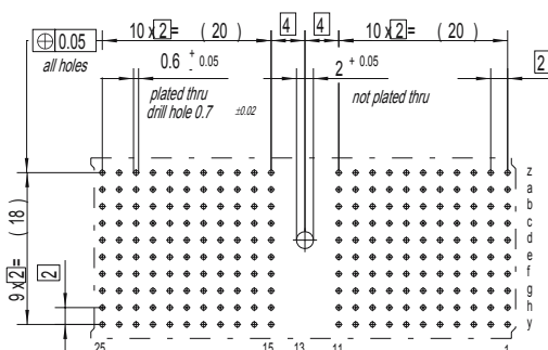
Lochbild fuer Leiterplatte (Bestueckungsseite)
