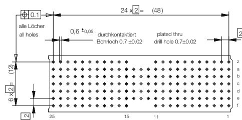
Lochbild fuer Leiterplatte (Bestueckungsseite)
