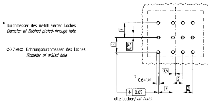
Lochbild für Leiterplatte / Board hole pattern
