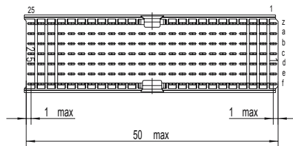
Lochbild fuer Leiterplatte (Bestueckungsseite)
