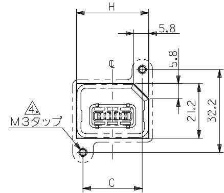
パネル取り付け穴推奨寸法 RECOMMENDED PANEL OPENING
