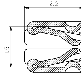
SECTION A-A (SCALE 20-1)
