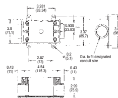
Type FDC
