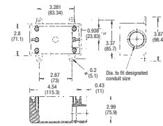
Type FDE
